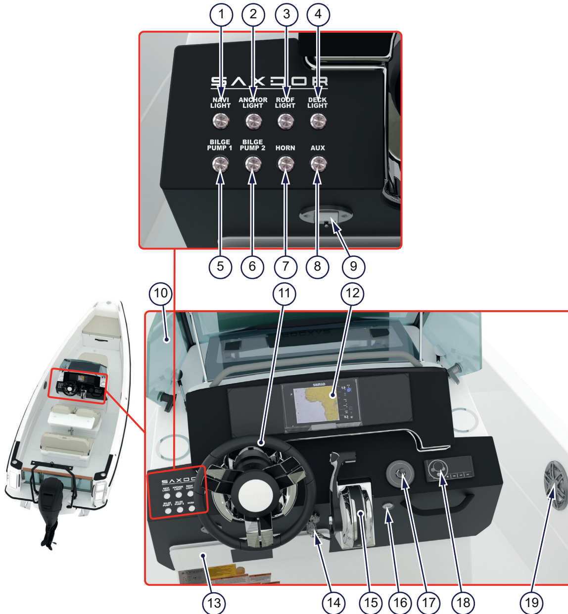
Kuva 4.7 - Ohjauspisteen hallintalaitteet
