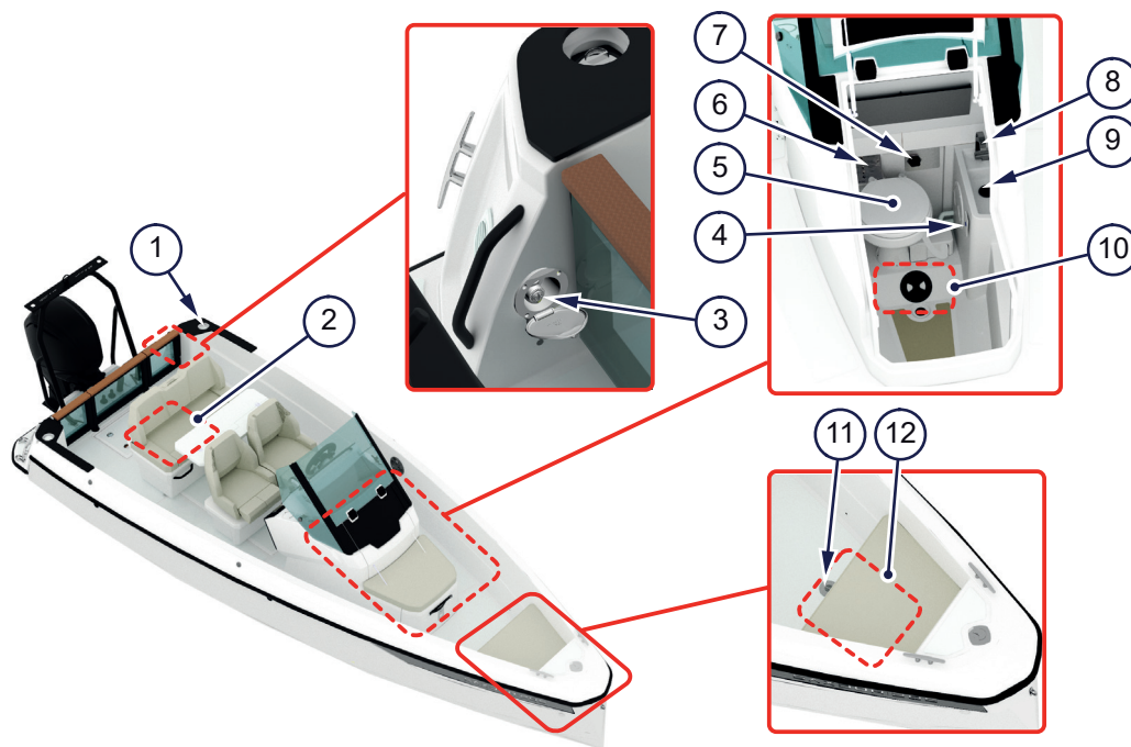
Kuva 5.5 - Makea- ja jätevesijärjestelmät
