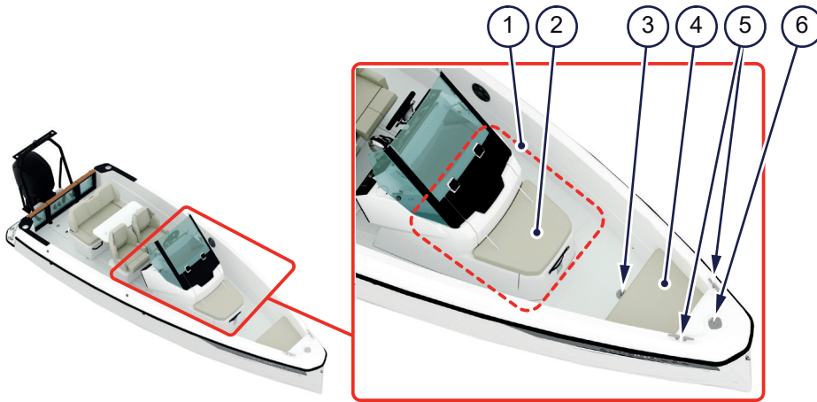
Kuva 4.2 - Etukansi
