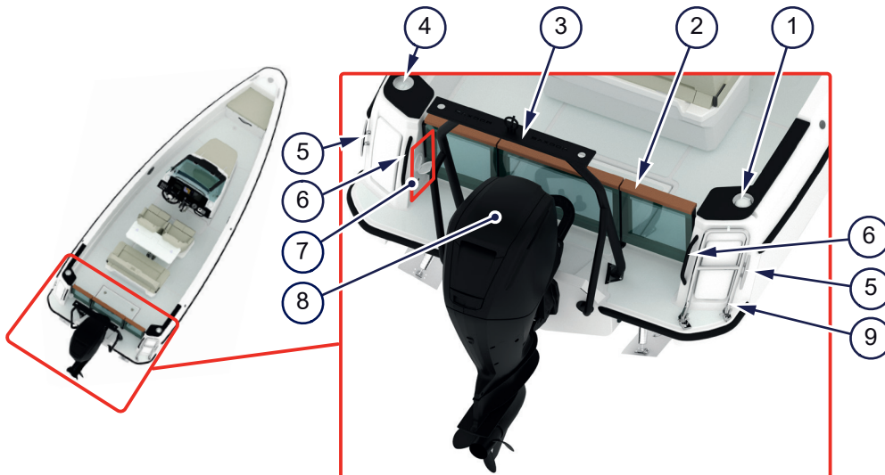
Kuva 4.5 - Uimatasanne
