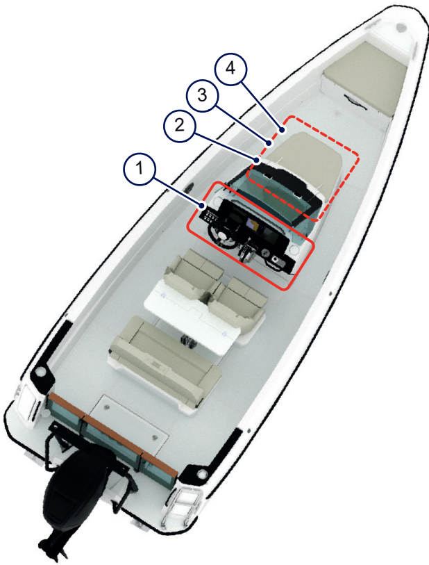
Kuva 4.6 - Käyttäjän hallintalaitteet
